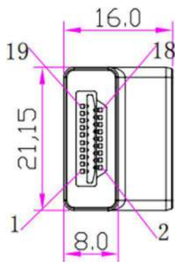
HDMI/AM
