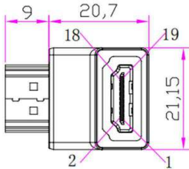
HDMI/AF
