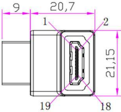
HDMI/AF
